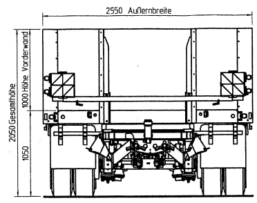
Schnitt A-A
