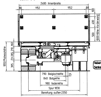
Schnitt C-C
