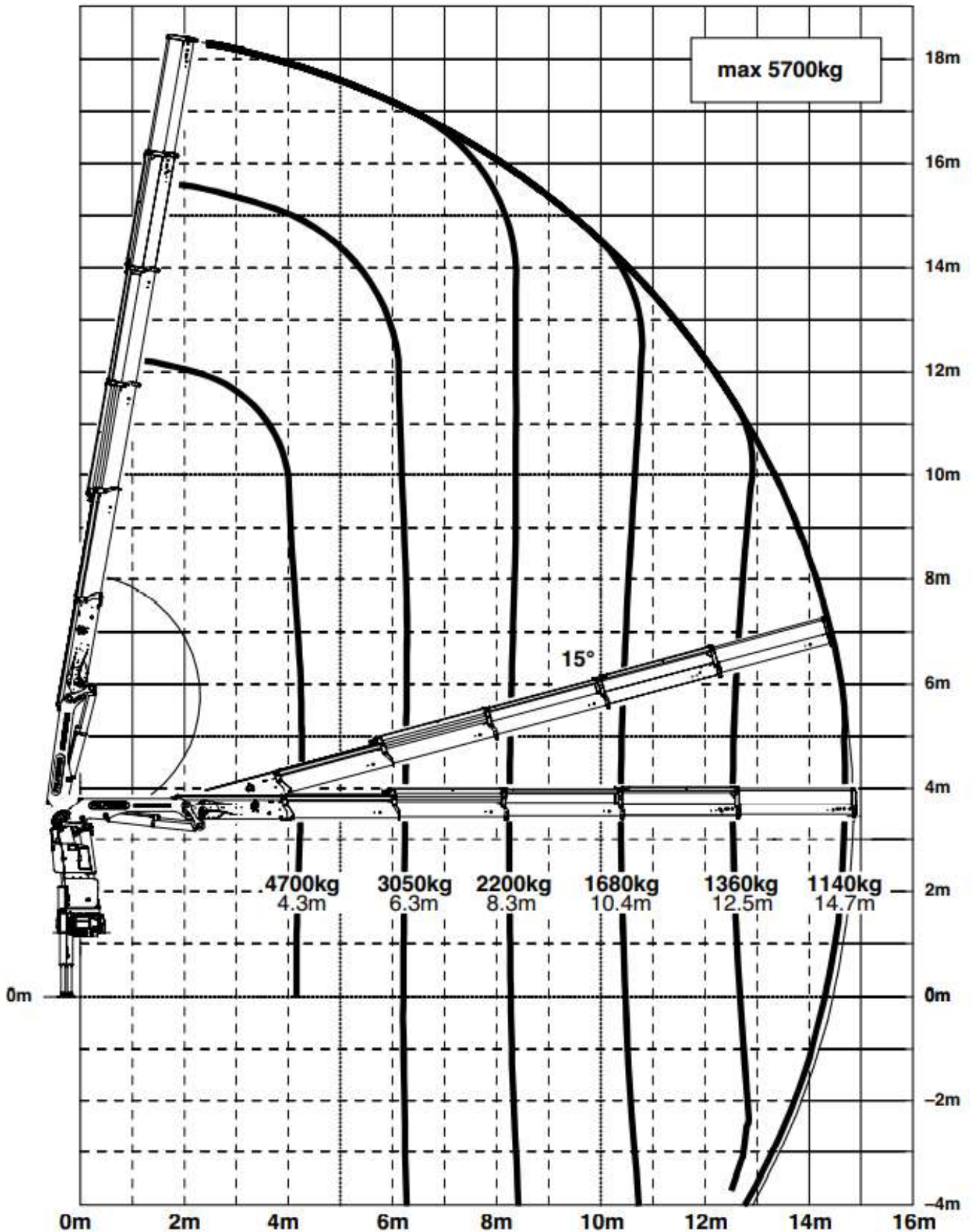
LKW 4-Achs-Kipperfahrzeug & Ladekran 23 m/to (variabel mit Greifer, Anhänger & Tieflader)
