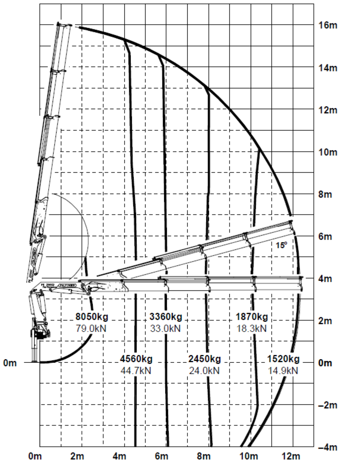
LKW 4-Achs-Kipperfahrzeug & Ladekran 23 m/to (variabel mit Greifer, Anhänger & Tieflader)
