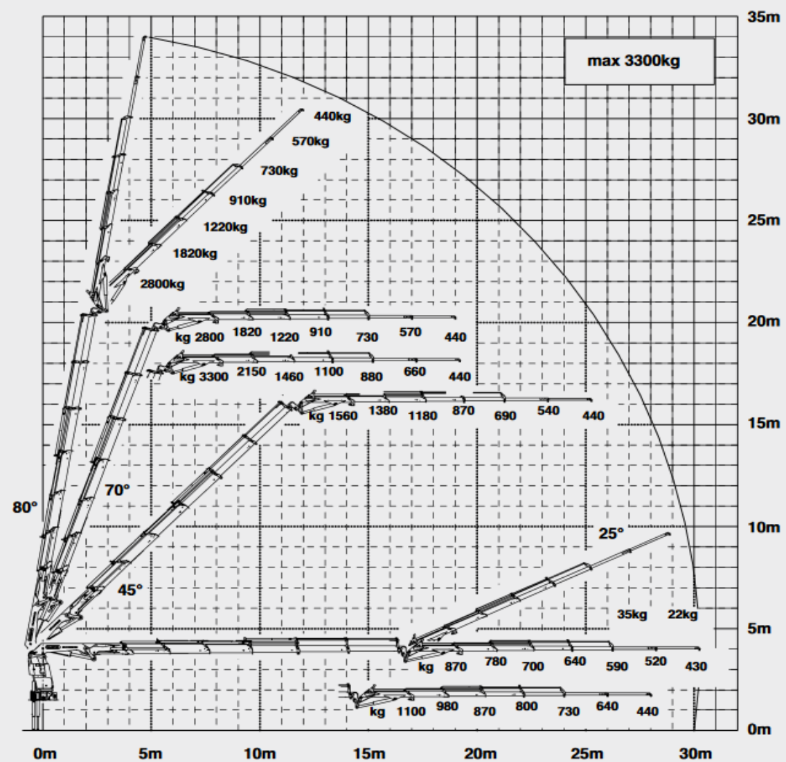
LKW 4- Achser & Ladekran 42 m/to + Jib (variabel mit Greifer & Tieflader)
