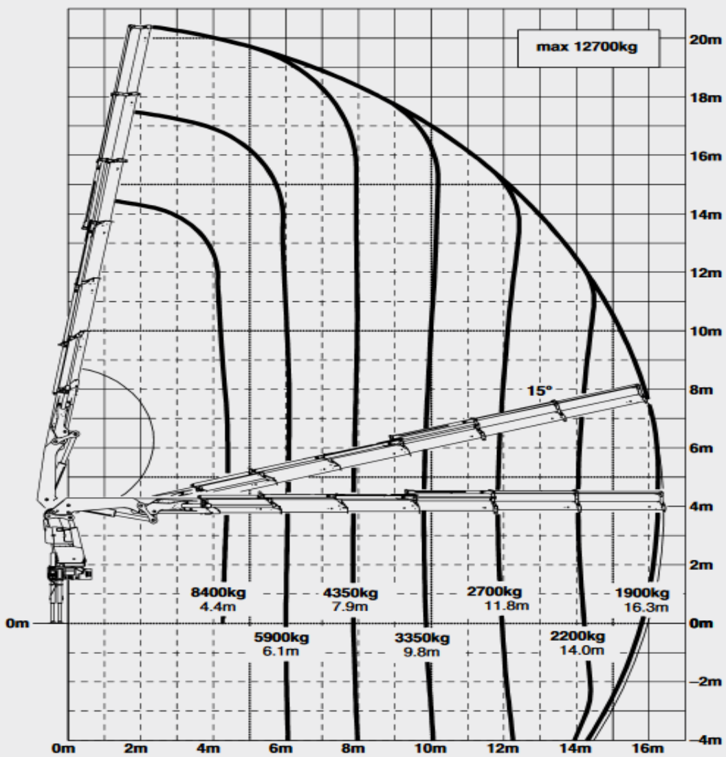
LKW 4- Achser & Ladekran 42 m/to + Jib (variabel mit Greifer & Tieflader)
